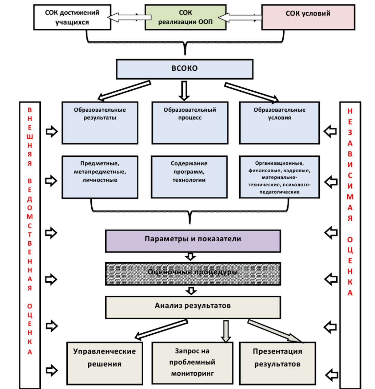
Рис. 1 – Структура ВСОКО
